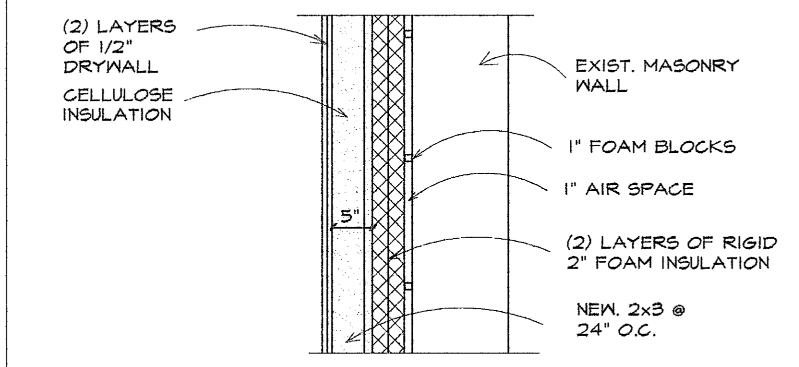
8 SECTION A-4 SCALE: 1" = 1'-0"
