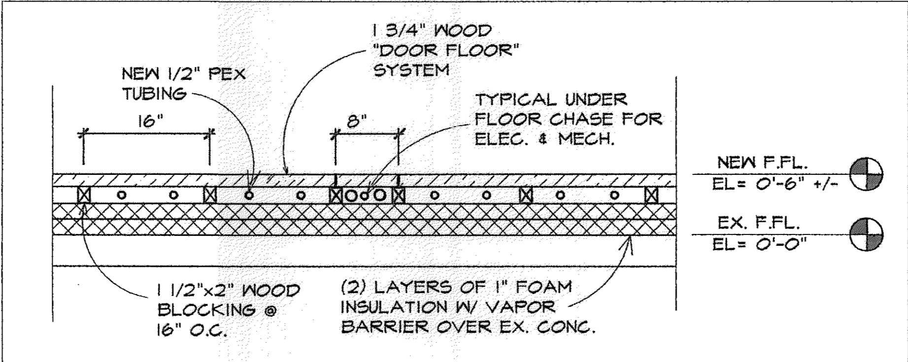
9 SECTION A-4 SCALE: 1" = 1'-0"
